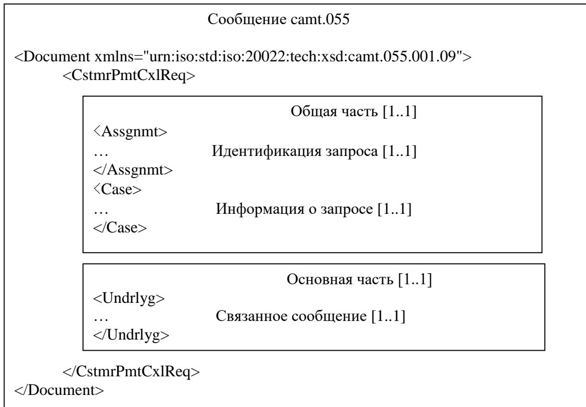
Рисунок 1 – Структура сообщения camt.055
