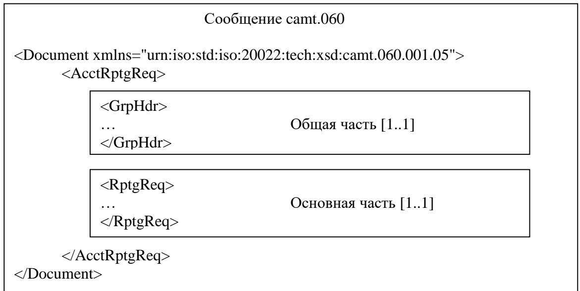
Рисунок 1 – Структура сообщения camt.060
