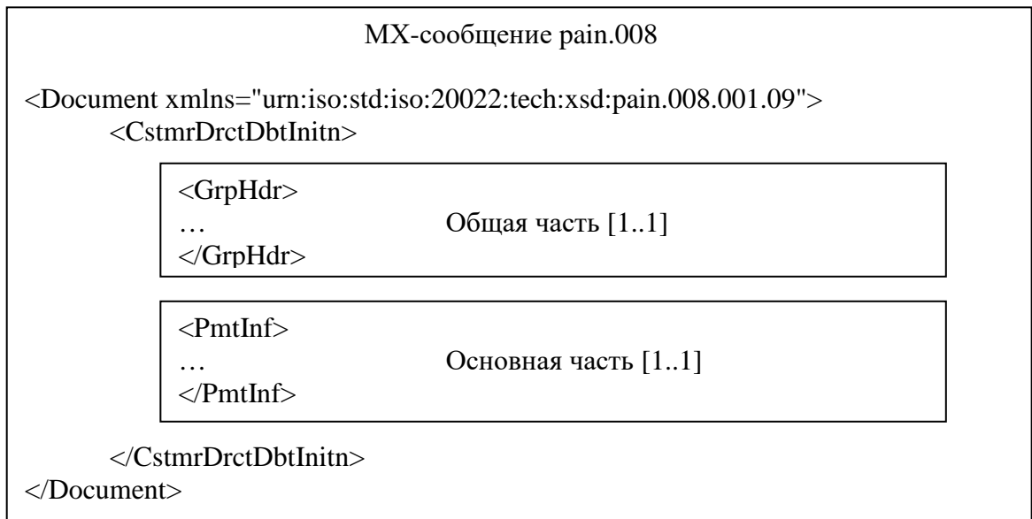
Рисунок 1 – Структура МХ-сообщения pain.008
