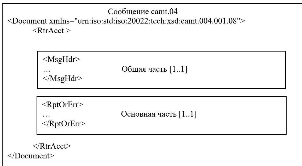
Рисунок 1 – Структура сообщения camt.004
