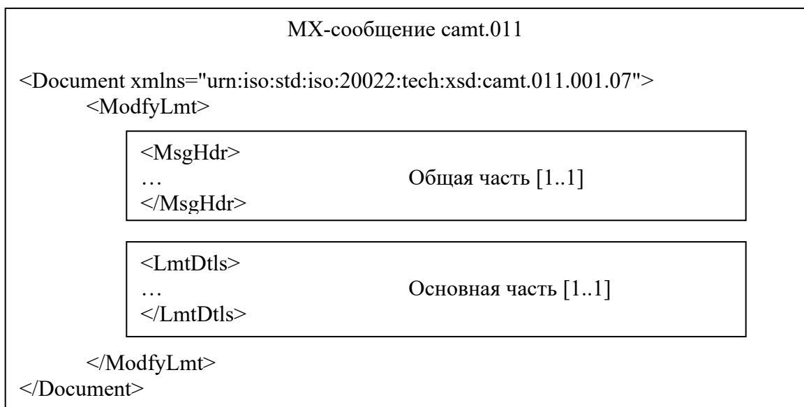
Рисунок 1 – Структура МХ-сообщения camt.011
