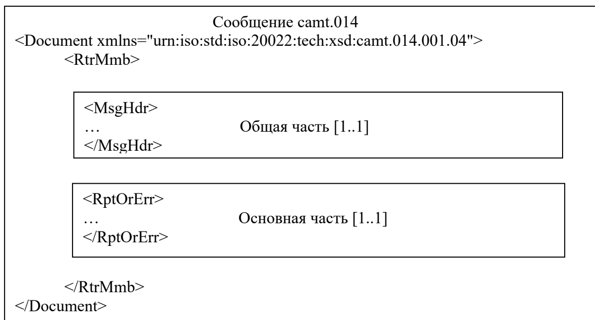
Рисунок 1 – Структура сообщения camt.014
