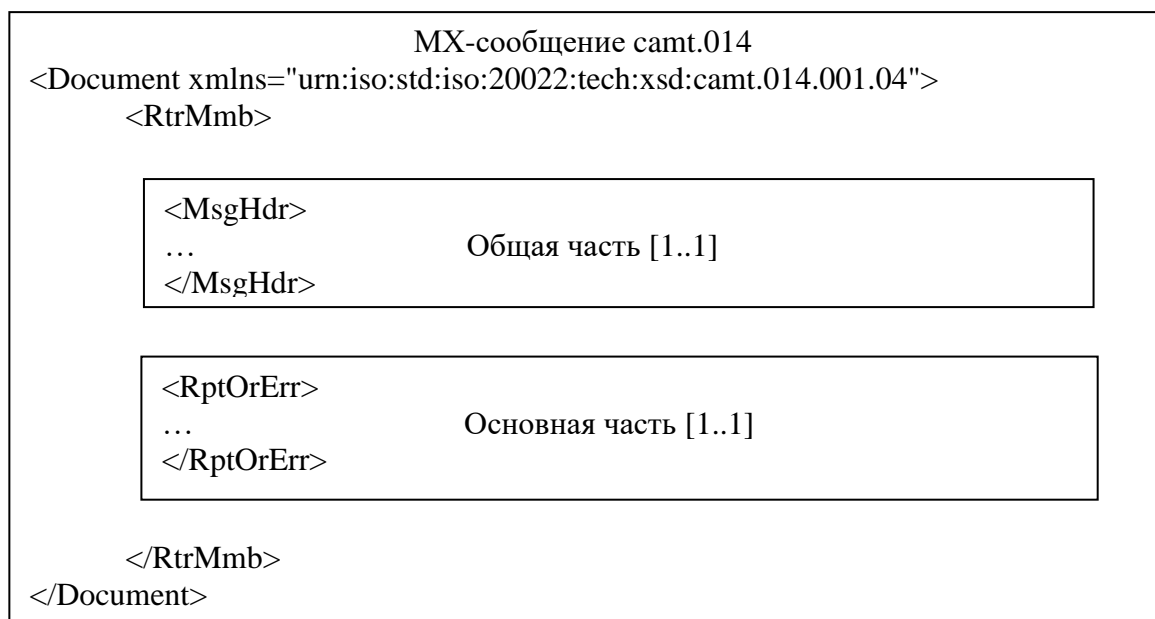
Рисунок 1 – Структура МХ-сообщения camt.014
