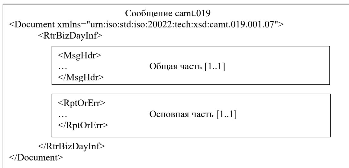
Рисунок 1 – Структура сообщения camt.019
