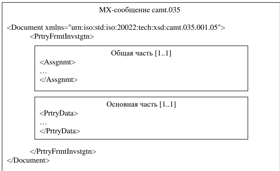
Рисунок 1 – Структура МХ-сообщения camt.035 подтип 09
