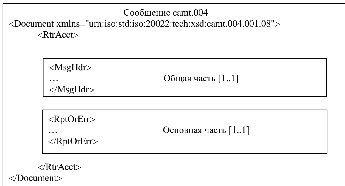
Рисунок 1 – Структура сообщения camt.004
