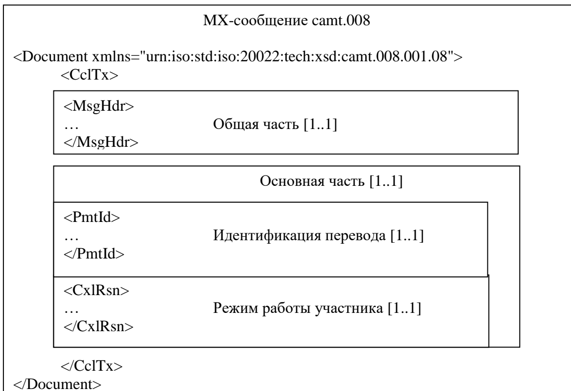
Рисунок 1 – Структура МХ-сообщения camt.008
