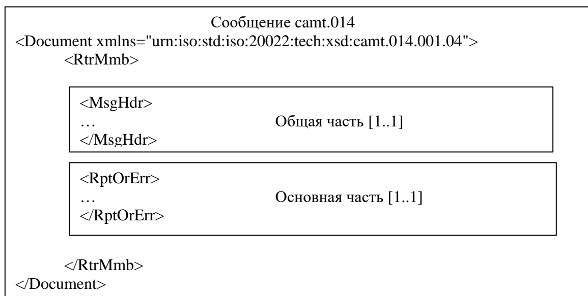
Рисунок 1 – Структура сообщения camt.014
