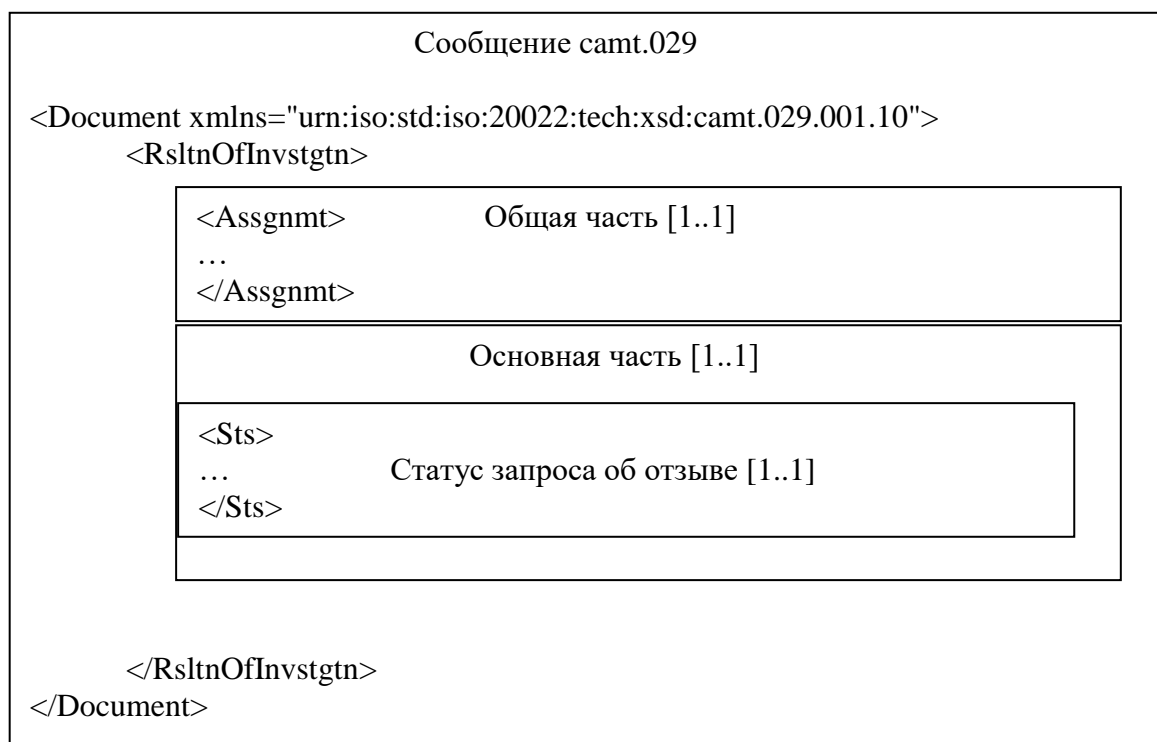
Рисунок 1 – Структура сообщения camt.029
