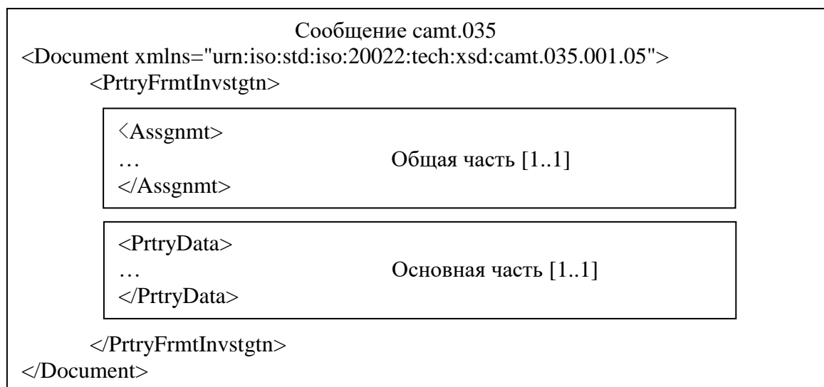
Рисунок 1 – Структура сообщения camt.035
