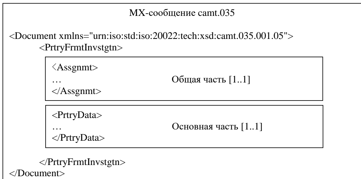
Рисунок 1 – Структура МХ-сообщение camt.035
