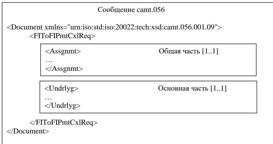
Рисунок 1 – Структура сообщения camt.056
