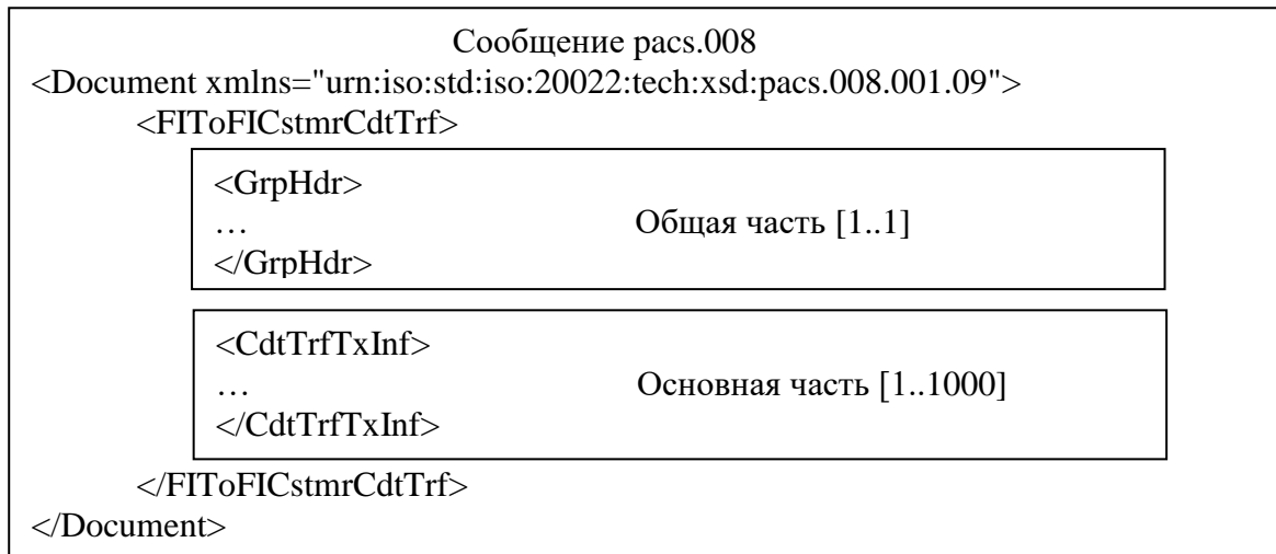
Рисунок 1 – Структура сообщения расс.008
