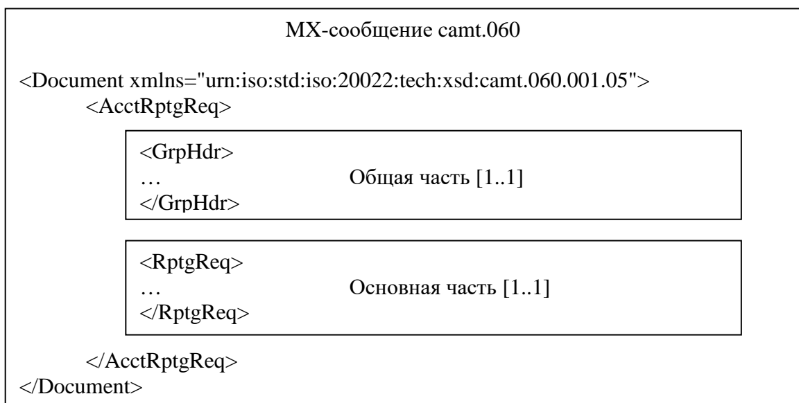
Рисунок 1 – Структура МХ-сообщения camt.060
