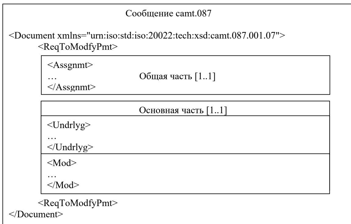
Рисунок 1 – Структура сообщения camt.087
